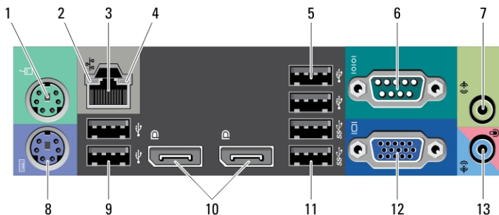
Figur 3. Minitower og desktop set fra bagpanel
