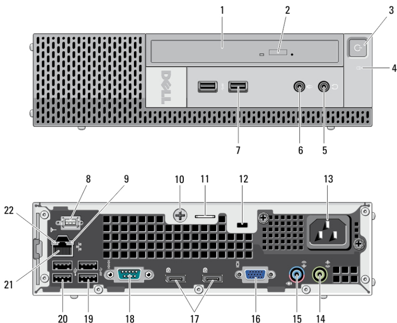
Figur 6. Ultra Small Form Factor set forfra og bagfra
